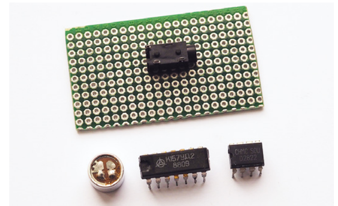
ШАГ 1. Приготовьте основные детали для сборки стетоскопа: электретный микрофон, микросхемы К157УД2 и TDA2822M, разъем для наушников, макетную плату, радиодетали и паяльник (не показаны).
