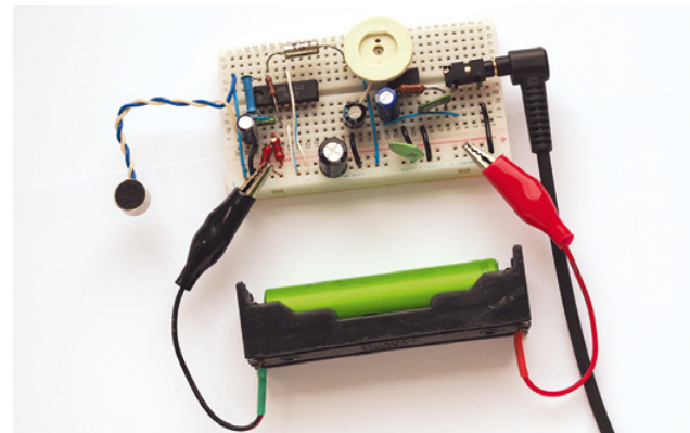
ШАГ 3. Подберите резистор R1 так, чтобы напряжение на выводе 13 операционного усилителя было равно половине напряжения питания. Добейтесь нужной чувствительности, подобрав значение R4.
