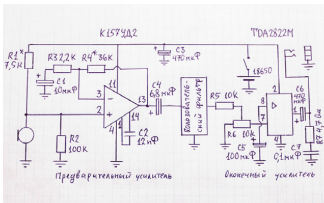
ШАГ 2. Соберите схему на беспаячной макетной плате. Неполарные конденсаторы C2 и C7 должны быть керамическими. Размещайте их как можно ближе к интегральным микросхемам.
